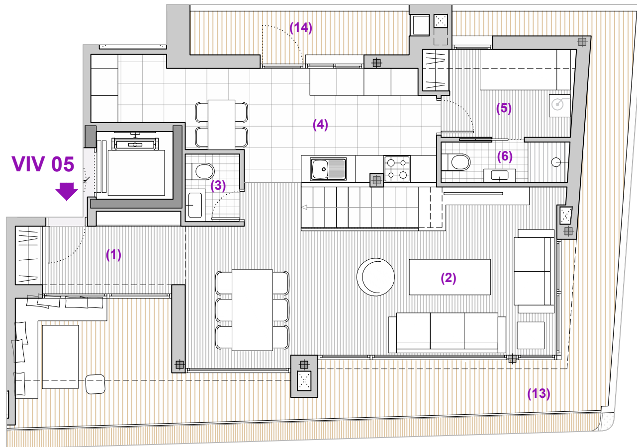
PLANTA TERCERA
